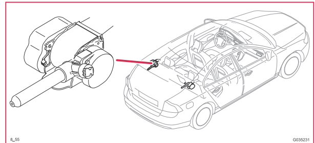
8/55 Zünder Gurtstraffer hinten links
