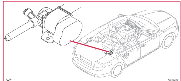
8/56 Zünder Gurtstraffer hinten rechts
