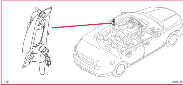
8/33 Zünder Gurtstraffer Fahrer
