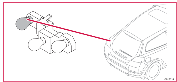
10/54 Blinker hinten links, C30
