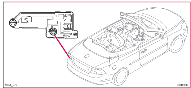
10/54 Blinker hinten links, C70
