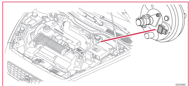
7/160 Bremsvakuumgeber
