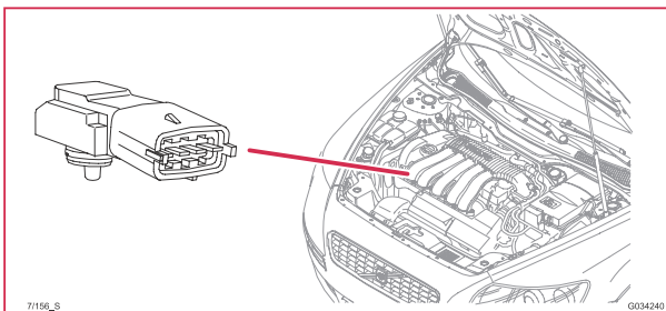
7/156 Druck- und Temperurgeber Kraftstoff, 5-Cyl.
