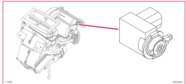
7/159 Luftqualitätssensor (AQS)
