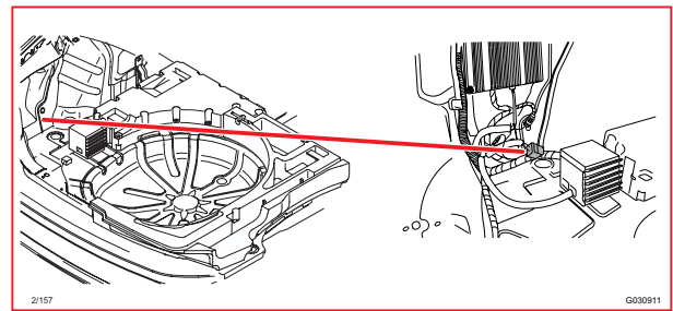
2/157 Relais Basslautsprechersteuergerät
