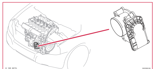
6/120 Drosselklappeneinheit, 6-Zyl.
