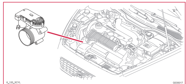
6/120 Drosselklappeneinheit, 5-Zyl.
